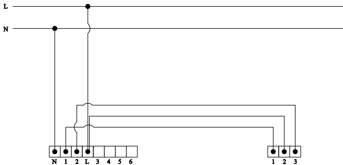
Limodor LF/M 100/40 típusú kétfokozatú kisventilátor
