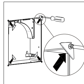
A ventilátorházat a kivágott falszerkezetbe betenni
